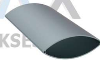
Güneş Kırıcı Profili Ürün Kodu: 2596 Ağırlık kg/m: 0,618 (30 x 80 x 1,3mm)
